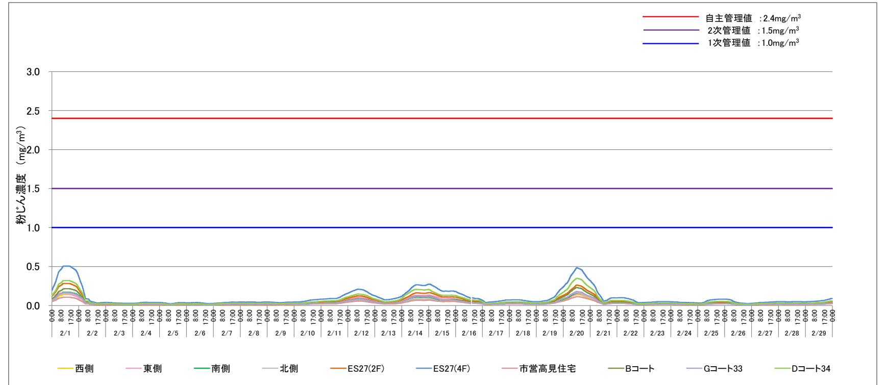
2024.2月度 粉じん濃度24時間移動平均値 (○:管理値超過なし、■:1次管理値超過、▲:2次管理値超過、×:自主管理値超過、-:データの欠測)
